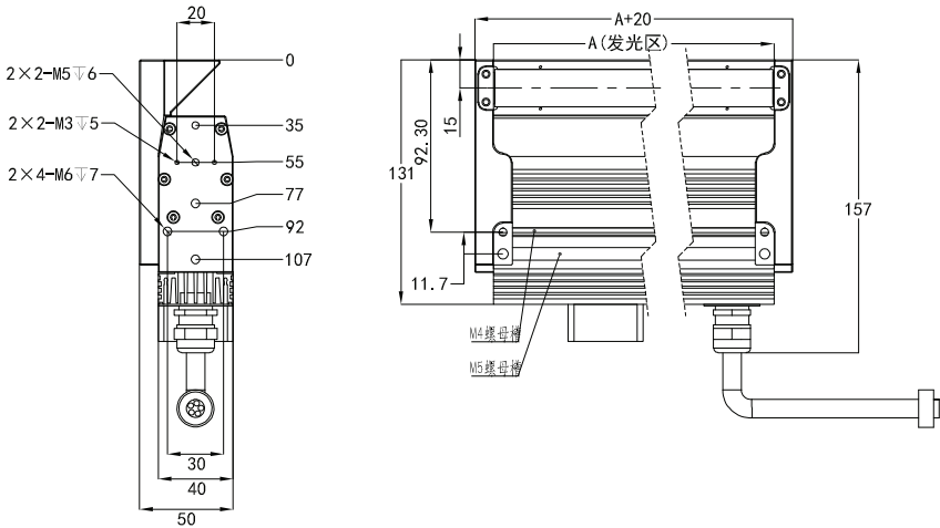
NORLEX-HLCL3-A同轴线性光源
