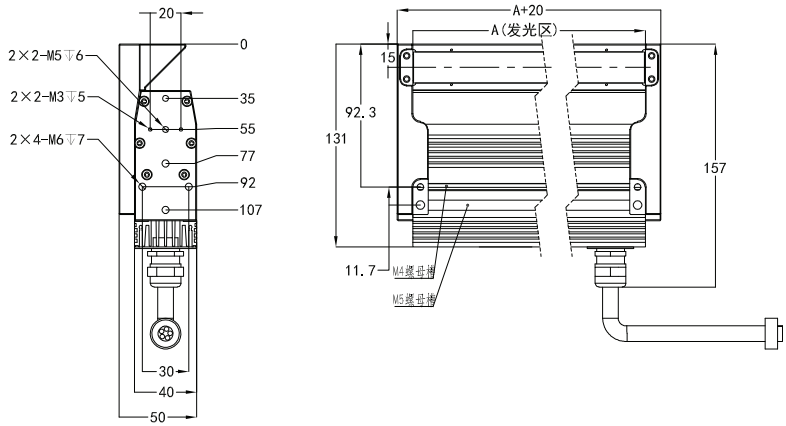
NORLEX-HLCL3-A同轴线性光源
