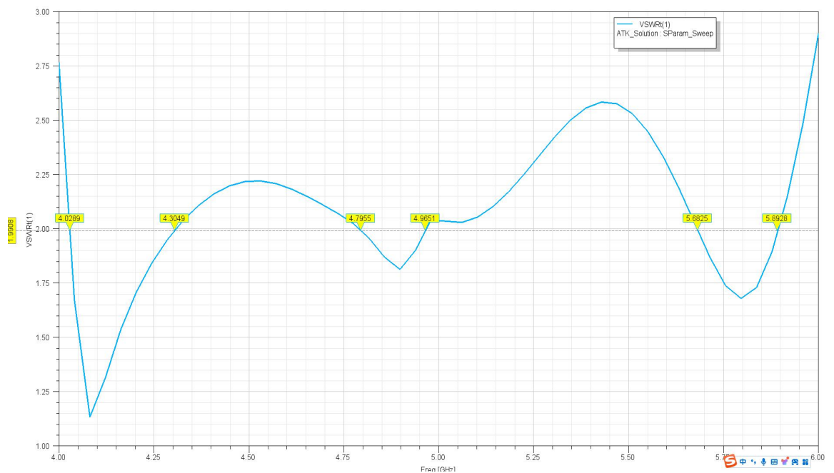
图 2-2 天线驻波比
