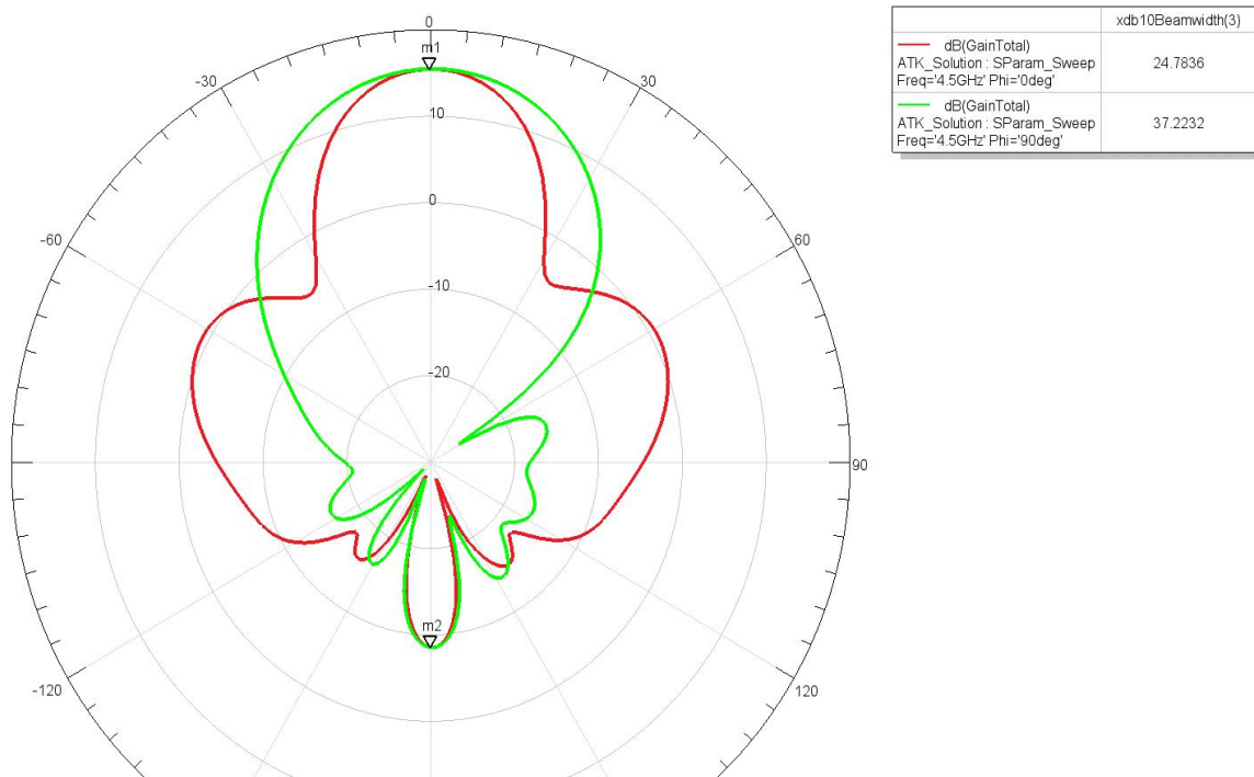
图 2-5 2D 天线方向图 4.5GHz
