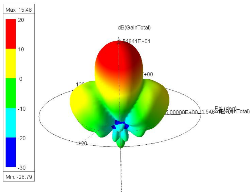
图 2-3 天线 3D 方向图
