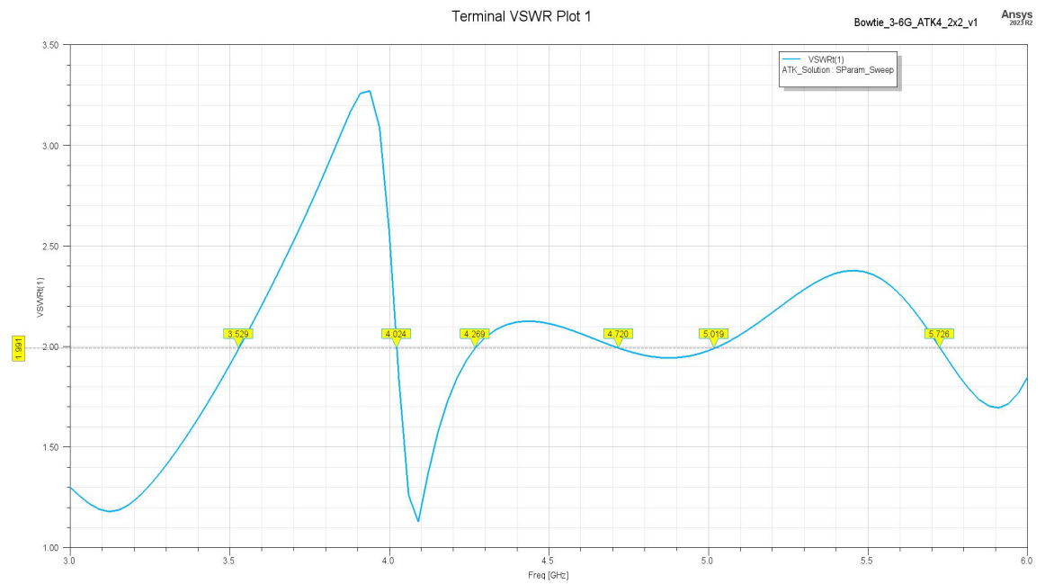
图 2-1 天线驻波比
