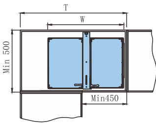
左开门或右开门共用示意图 Left or right is same one
