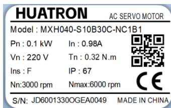
电机铭牌
