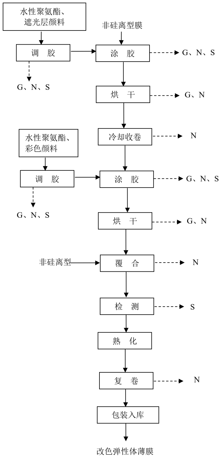
图2-4 改色弹性体薄膜生产工艺流程及产排污环节图
