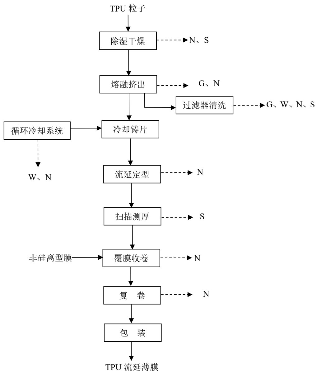
图2-2 TPU流延薄膜生产工艺流程及产排污环节图
