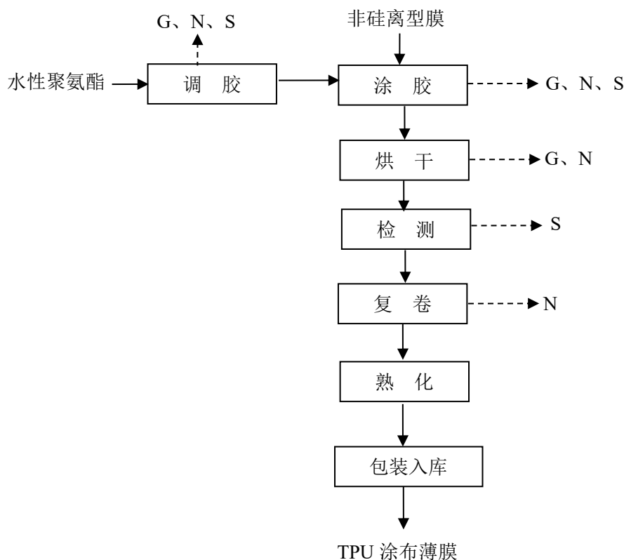
图 2-3 TPU 涂布薄膜生产工艺流程及产排污环节图
